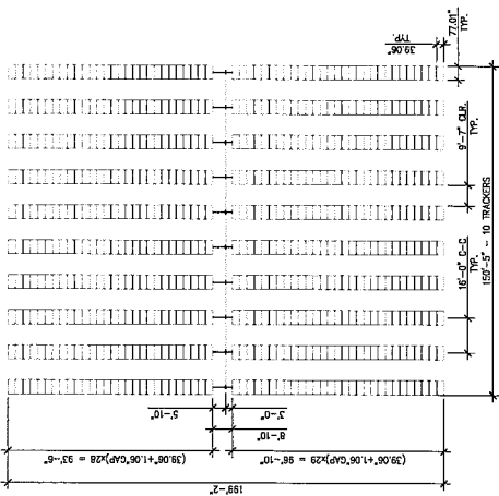
6 TYPE 6 SUB-ARRAY DETAIL SCALE: 1" = 30'-0" MODULE: JINGO 34
