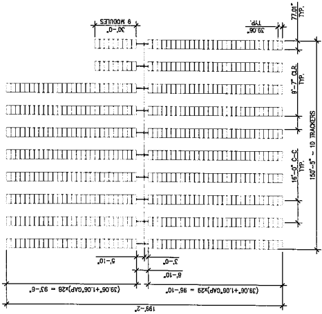
7 TYPE 7 SUB-ARRAY DETAIL SCALE: 1" = 30'-0" MODULE: JINGO 34
